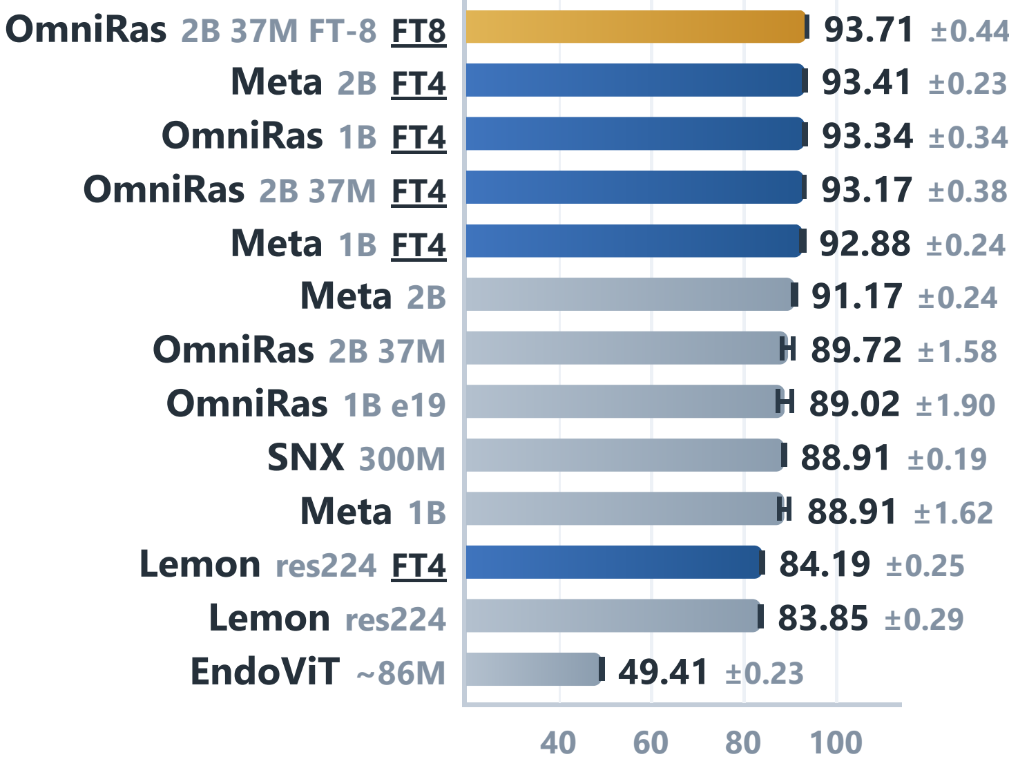
Tool mAP
